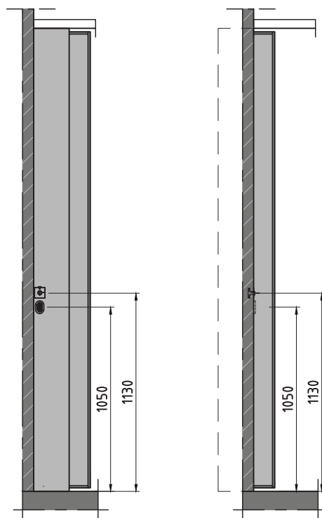
Telescopische wandlijst
