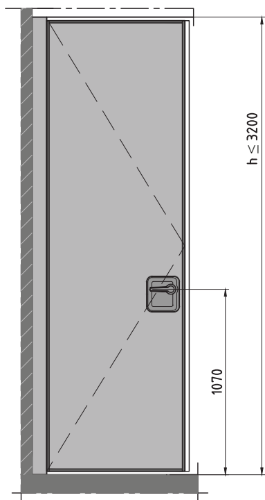
Communicatiepaneel
