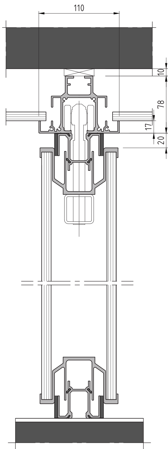
I-punts ophanging
