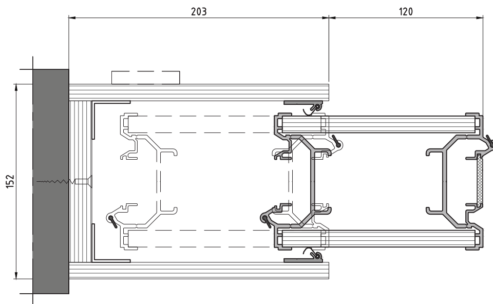
Detail telescopische wandlijst , opbouw
