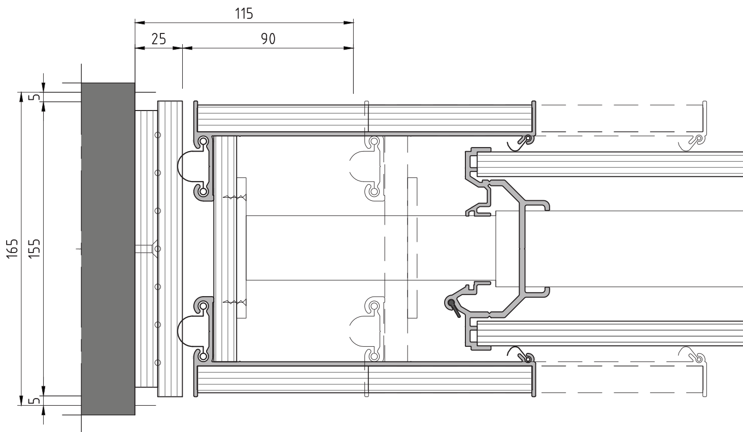
Detail telescoopzijde
